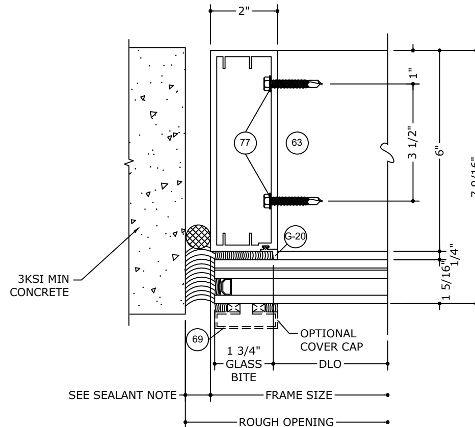
3.1 JAMB DETAIL (CONCRETE) N.T.S
