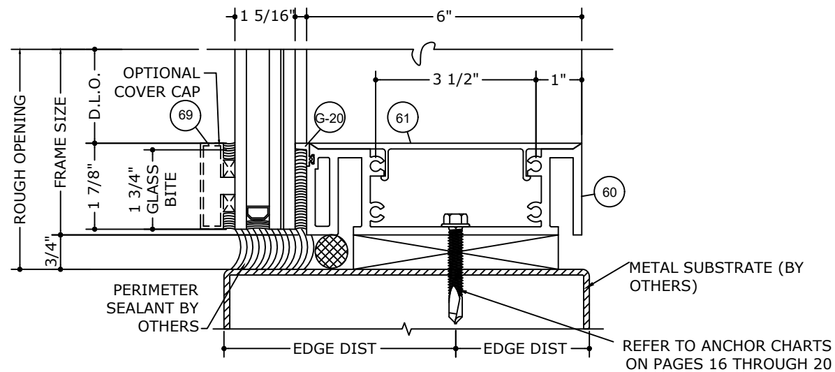
2.3 SILL DETAIL (METAL) N.T.S
