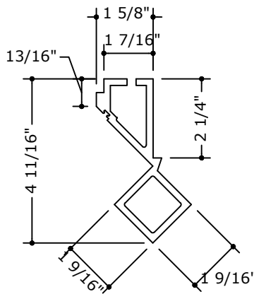
75 90° CORNER CAP
