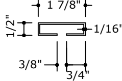
69 EXTERIOR CAP
