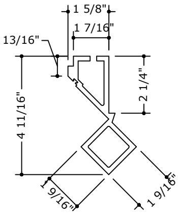
76 90° CORNER CAP
