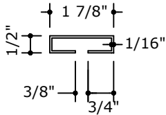
69 EXTERIOR CAP
